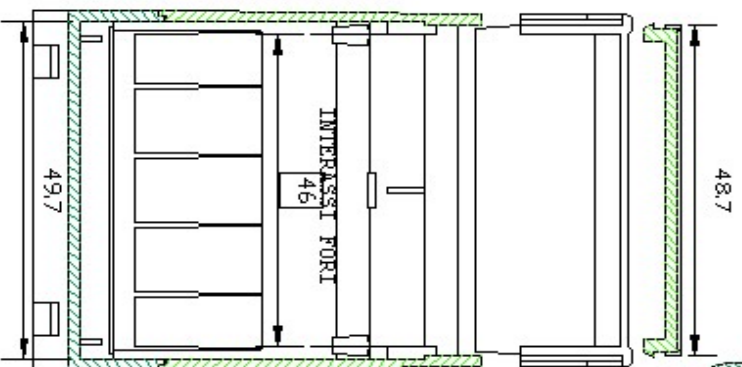
Sez. B-B
