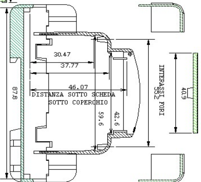
Sez. A-A
