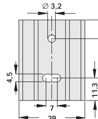
SK 145 37,5 TO 220
